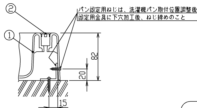
床固定部詳細(1:3)
